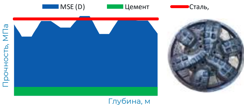
Диаграмма MSE по глубине относительно затрат энергии на разбуривание стали и цемента
